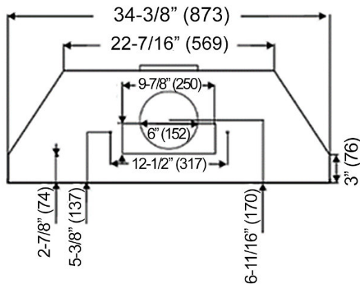
Vista Trasera
