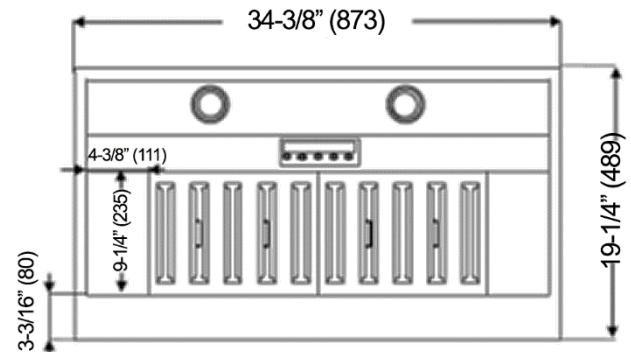
Vista Inferior
