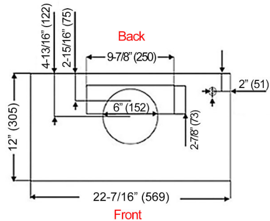
Vista Superior
